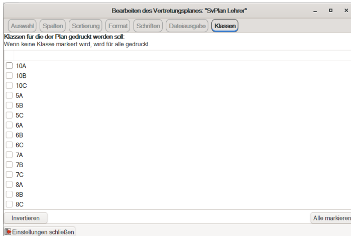
Abbildung 9.7: Klassenfilter
