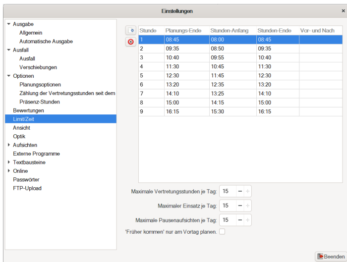
Abbildung 5.9: Einstellungen - Limit/Zeit
